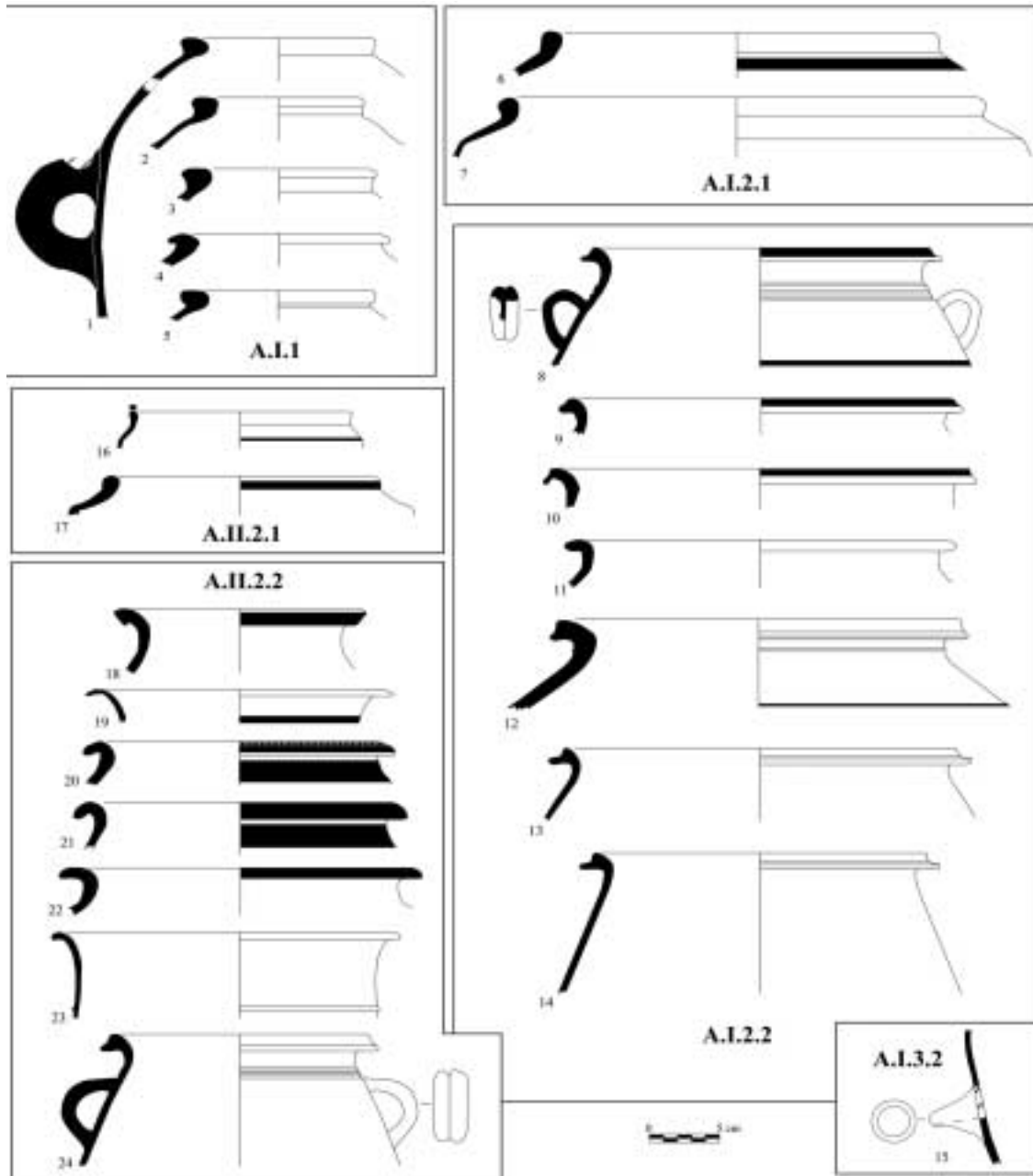
Fig. 8.- Tipologia ceràmica: 1-5, àmfores; 6-7, tenalles amb muscle; 8-14, tenalles sense muscle; 15, tenalla amb broc inferior; 16-17, tenalletes amb muscle; 18-24, tenalletes sense muscle.
